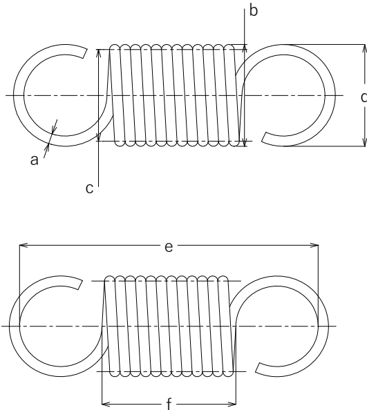
引きばね参考図
